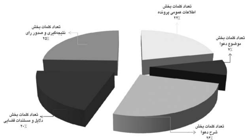
نمودار ۲-۵ فراوانی کمیت زبانی بخش‌های مختلف در خلاصه آرای ۵-۱
