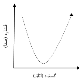
نمودار ۷: پیوند دو ساختار افزایشی و کاهشی ناهمسو
