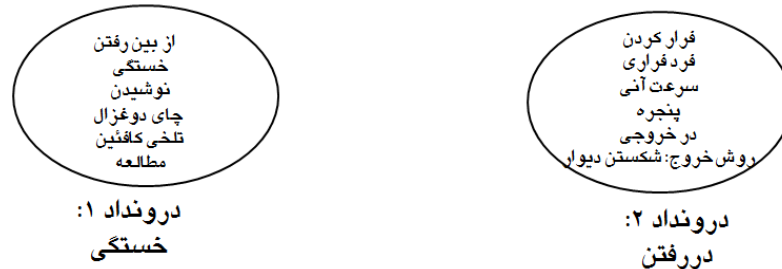
شکل ۴: درون‌داده‌های مثال ۴
