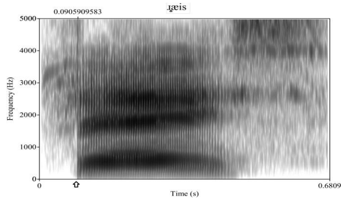
شکل ۶. طیف‌نگاشت واژه «رئیس» که در آن رآوا به صورت گونه سایشی بی‌واک تولید شده. Figure 6. Spectrogram of the word \text{ɹ̥ɪs} in which [\text{ɹ̥}] is produced as voiceless fricative
